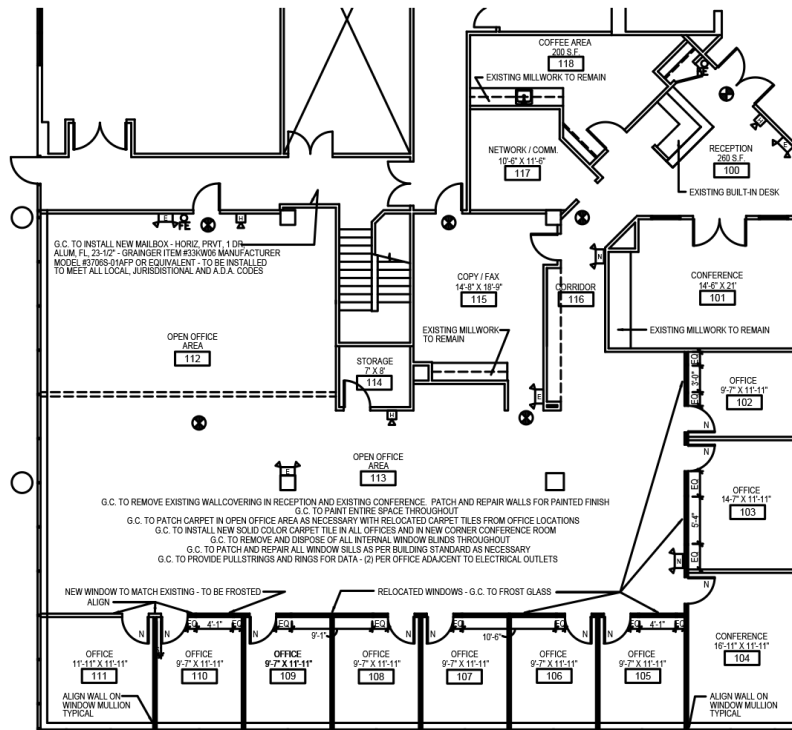
1 FLOOR PLAN SCALE: 1/8" = 1'-0"
